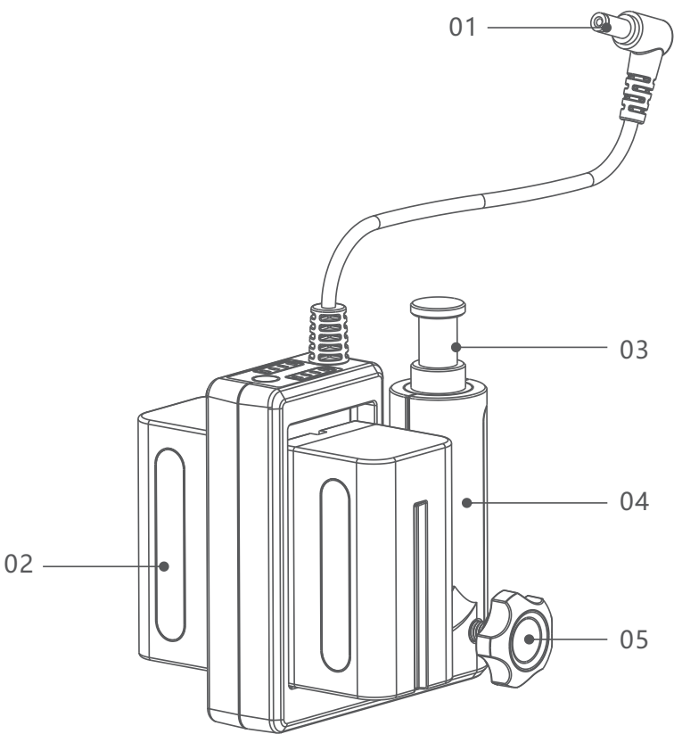
01 电源插头 02 电池（需要另购） 03 灯支架接头 04 手柄 05 安装锁紧旋钮
